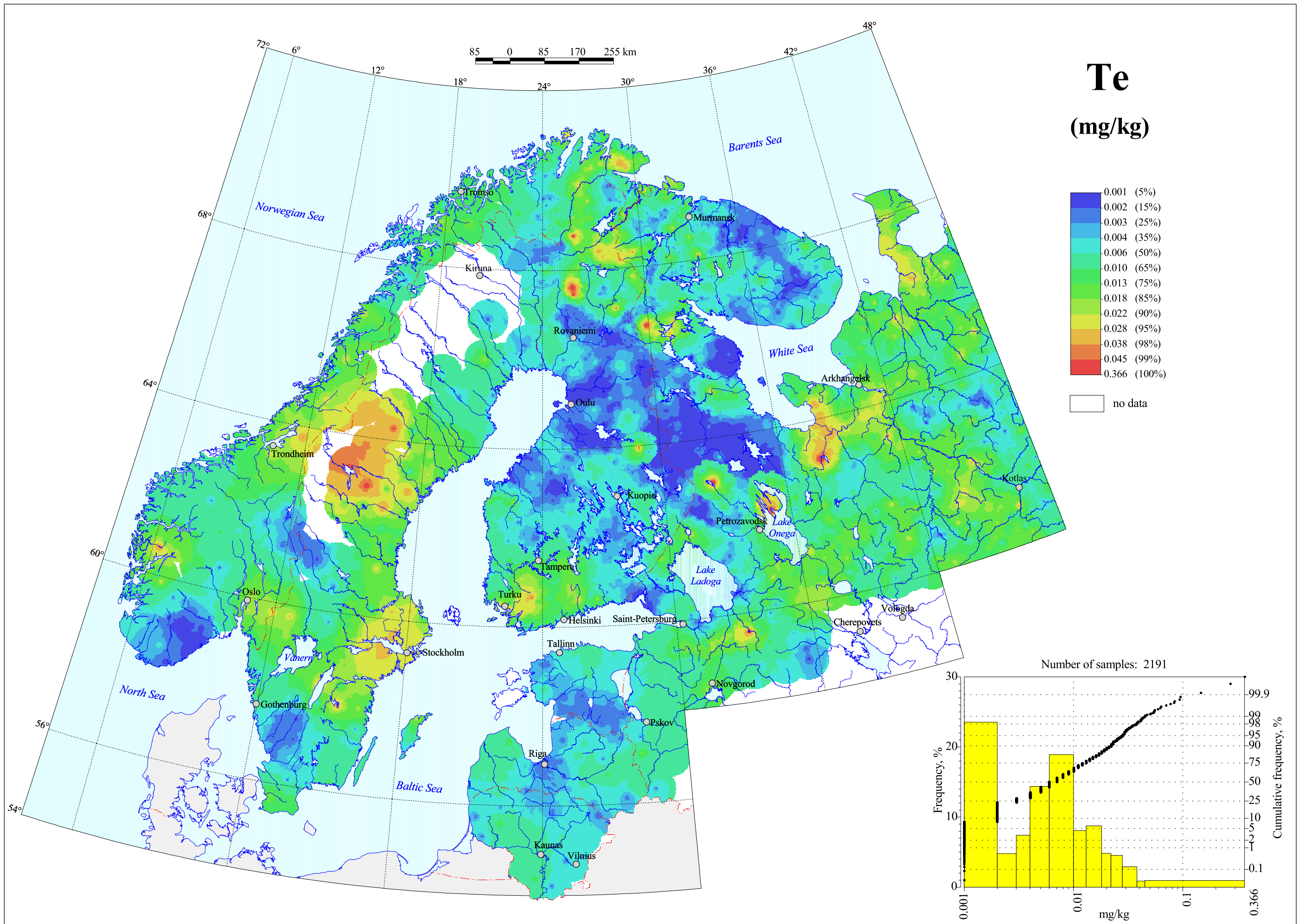
Tellurium in C-horizon, Grain Size <2 mm, Aqua regia Extraction
